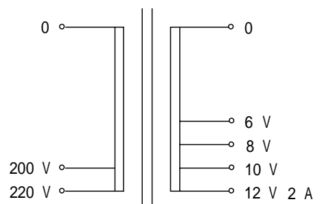
結線図
