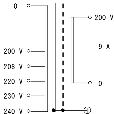
結線図
