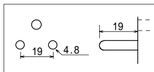
入力プラグ寸法
